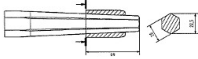
6-kt konisch
